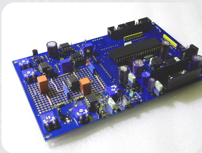
Eine Prüfplatine
